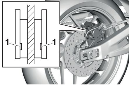
1. Fren balataları aşınma göstergesi
