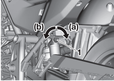
1. Sıkışma sönümlenme kuvveti ayarlama vidası
