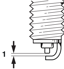
1. Buji aralığı
