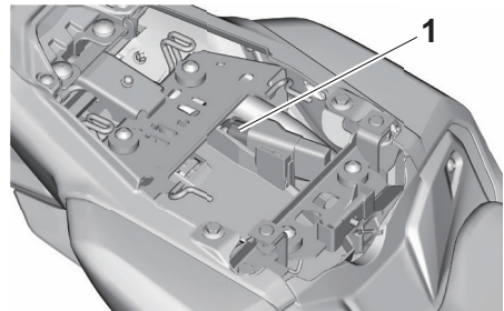
1. Teşhis konektörü
