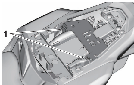
1. Kask tutucusu
