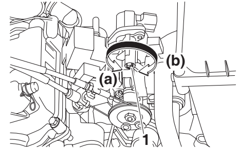
1. Rölantı ayar vidası
