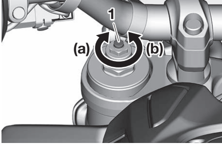
1. Sıkışma sönümlleme kuvveti ayarlama vidası
