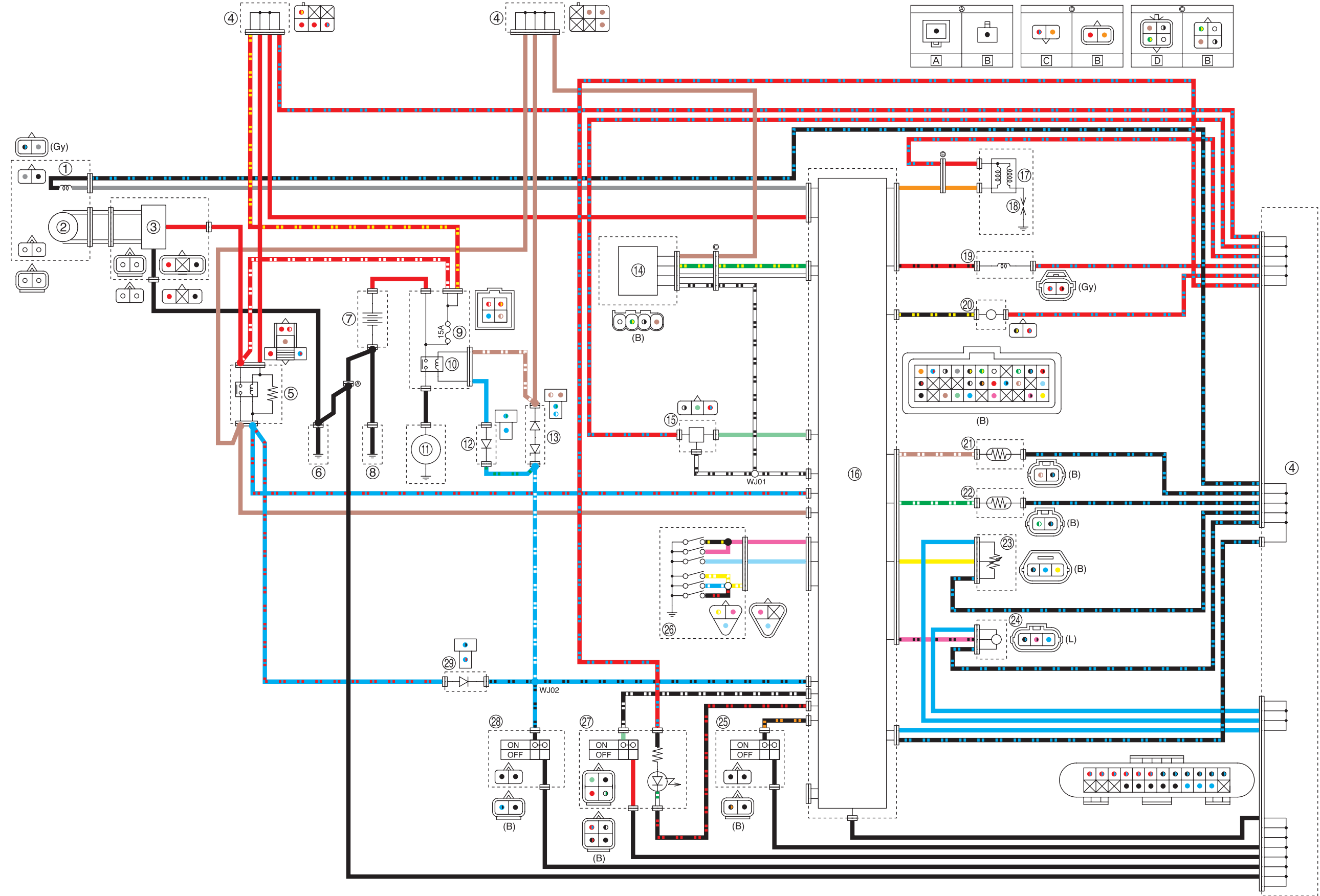
YZ250F/YZ250FP 2023 KABLO ŞEMASI
