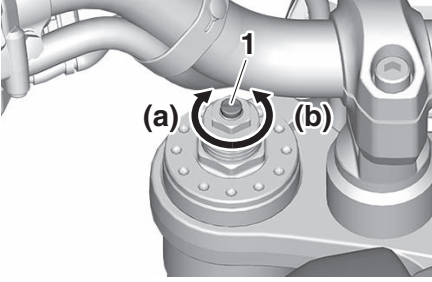
1. Sıkışma sönümlleme kuvveti ayar civatası (hızlı sıkışma sönümlmesi için)
