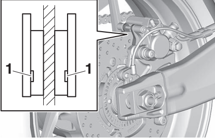
1. Fren balataları aşınma göstergesi oluđu
