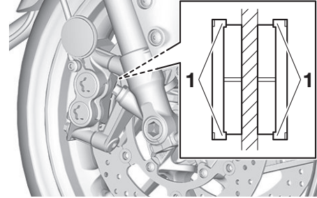
1. Fren balatası aşınma göstergesi
