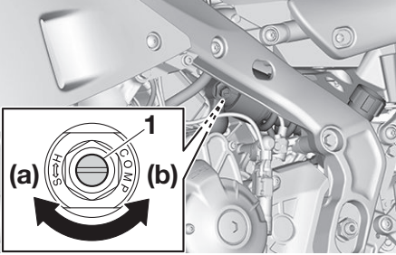
1. Yavaş sıkıştırma sönümleme kuvveti ayarlama vidası
