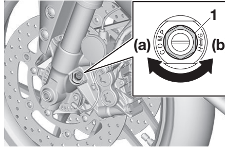
1. Hızlı sıkışma kuvveti ayar civatası
