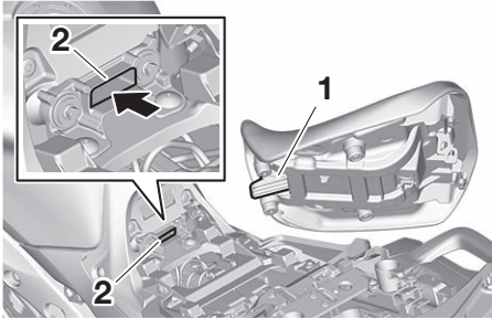
1. Çıkıntı 2. Sele tutucu B (yüksek konum için)
