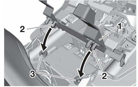
1. Sürücü selesi yükseklik konumu ayarlayıcısı 2. Çıkıntı 3. Gromet
