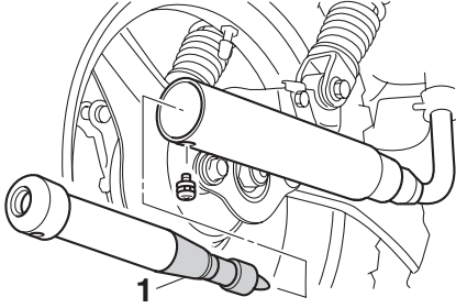
1. Kıvılcım önleyici
