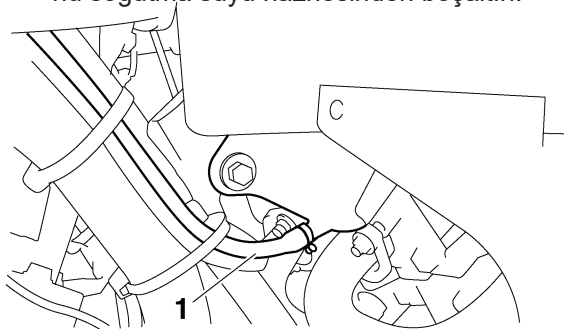
1. Soğutma suyu haznesi hortumu
