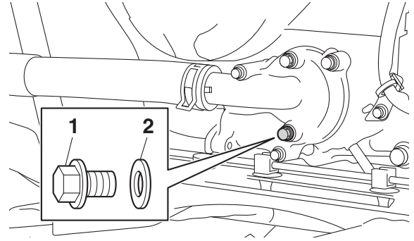
1. Soğutma suyu tahliye cıvatası
