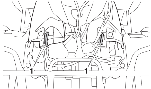
1. Hortum
