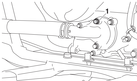
1. Su pompası hava boşaltma cıvatası
