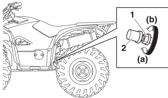
1. Arka fren lambası anahtarı ayarlama somunu
