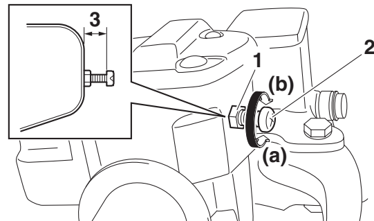
1. Kilit somunu
