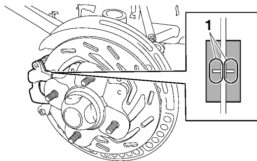
1. Aşınma gösterge oluşu
