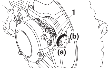
1. Arka fren kolu boşluğu ayar somunu
